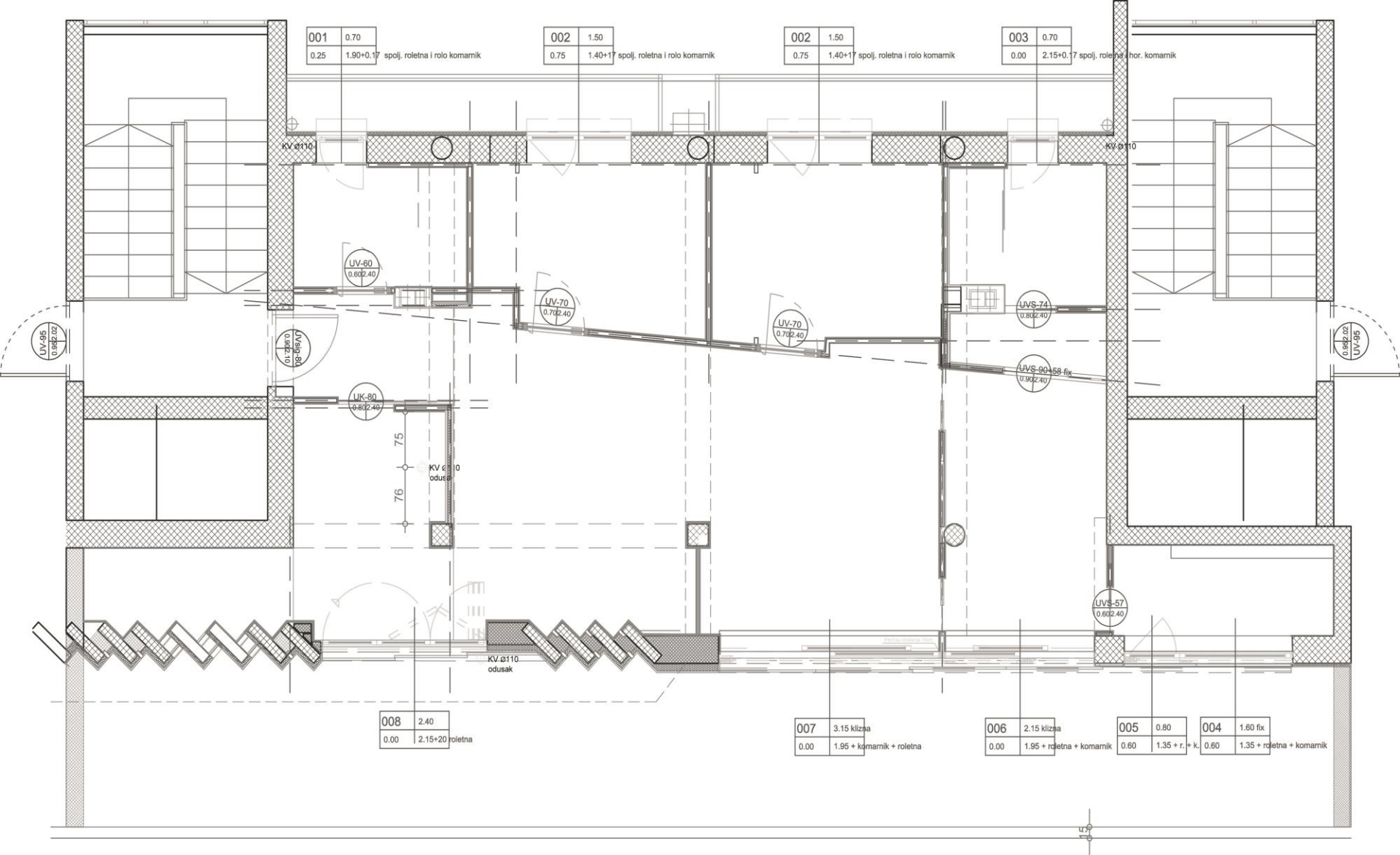
Пројекат ентеријера стамбеног простора у стамбено пословном објекту, Нови Сад, Кеј жртвава рације 4а Аутор- др Дубравка Ђукановић, диа
