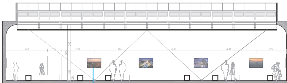
PRESEK A-A
